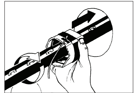
4.6 Um Kabel legen und in Kabelkanalzug einschieben.
