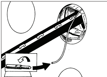
4.7 Füllschlauch der TDUX/ADE mit Schlauchadapter der Druckgasfüllvorrichtung verbinden.
