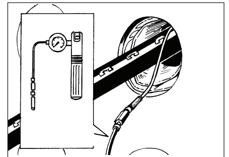
4.9 Füllen. Gebrauchsanleitung Druckgasfüllvorrichtung beachten.
